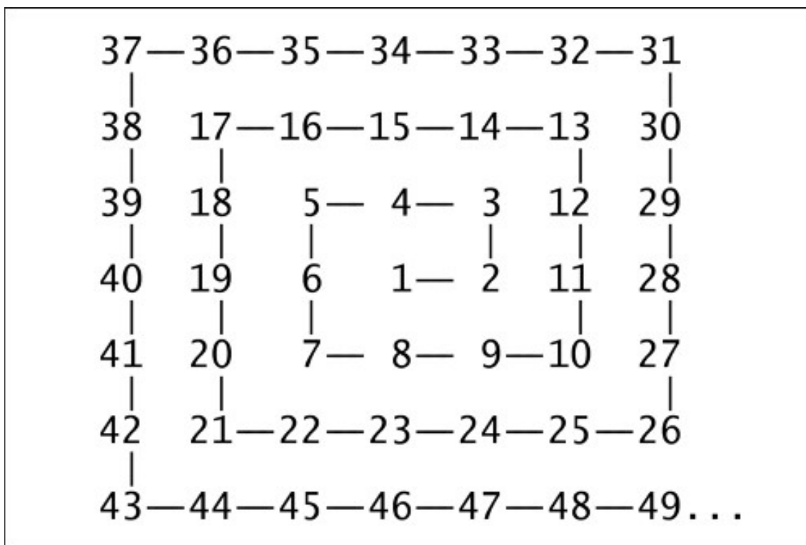
Liczby od 1 do 50 w układzie spirali Ulama
