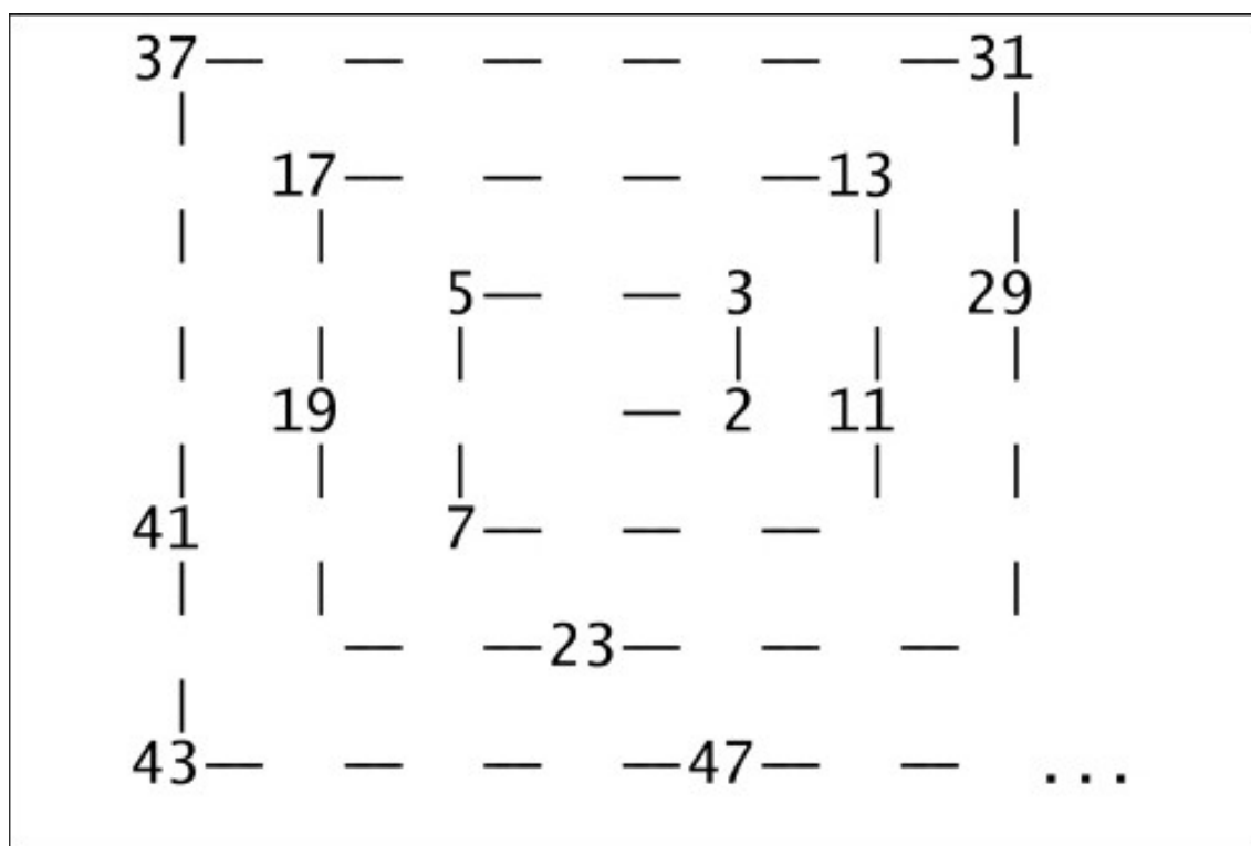
Liczby pierwsze od 1 do 50 w tym samym układzie
